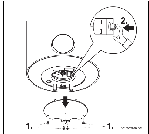
Sl. 10 Sigurnosni termostat
